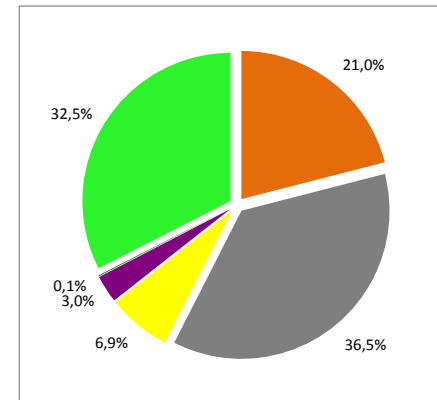
Verbleibender Energieträgermix
