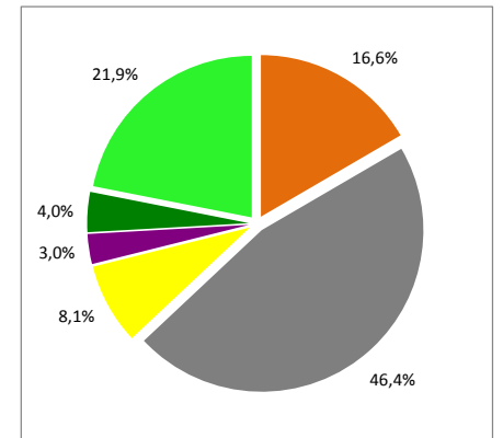
Energieträgermix Deutschland
