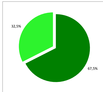
Energieträgermix Ökostromprodukt*
